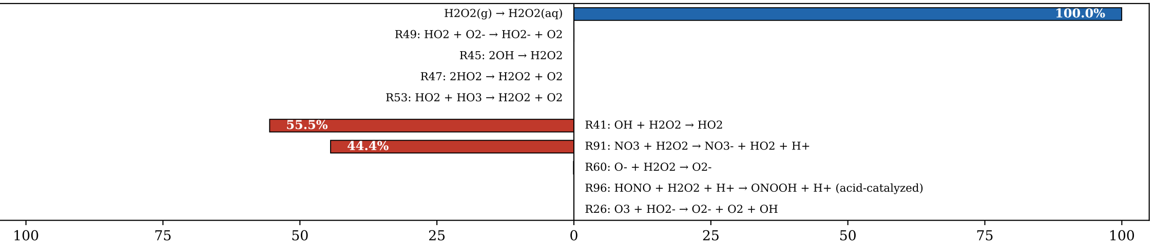
(d) \text{H}_2\text{O}_2 ( \Sigma\text{src} = 1.06\text{e-}08 \text{ M/s} )
